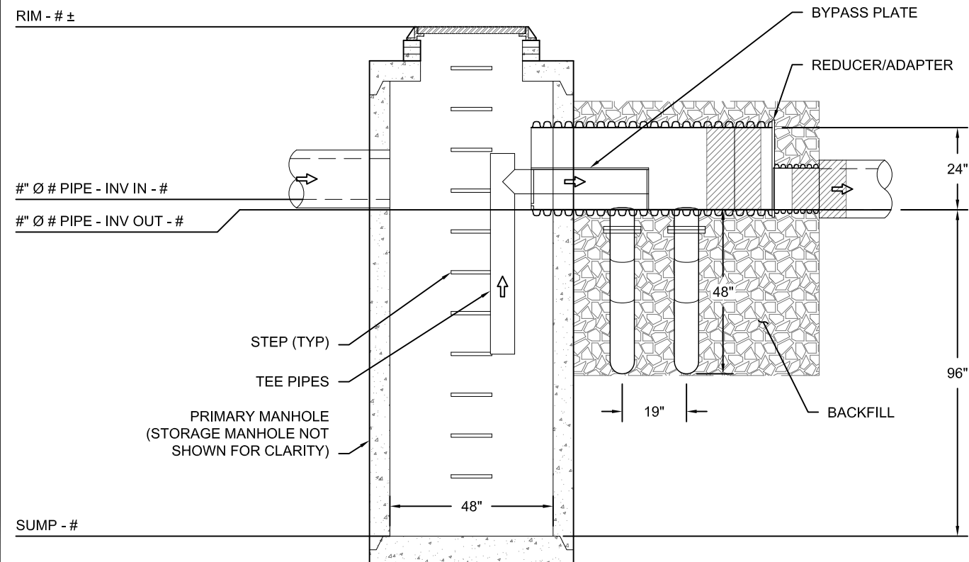
PROFILE A-A
