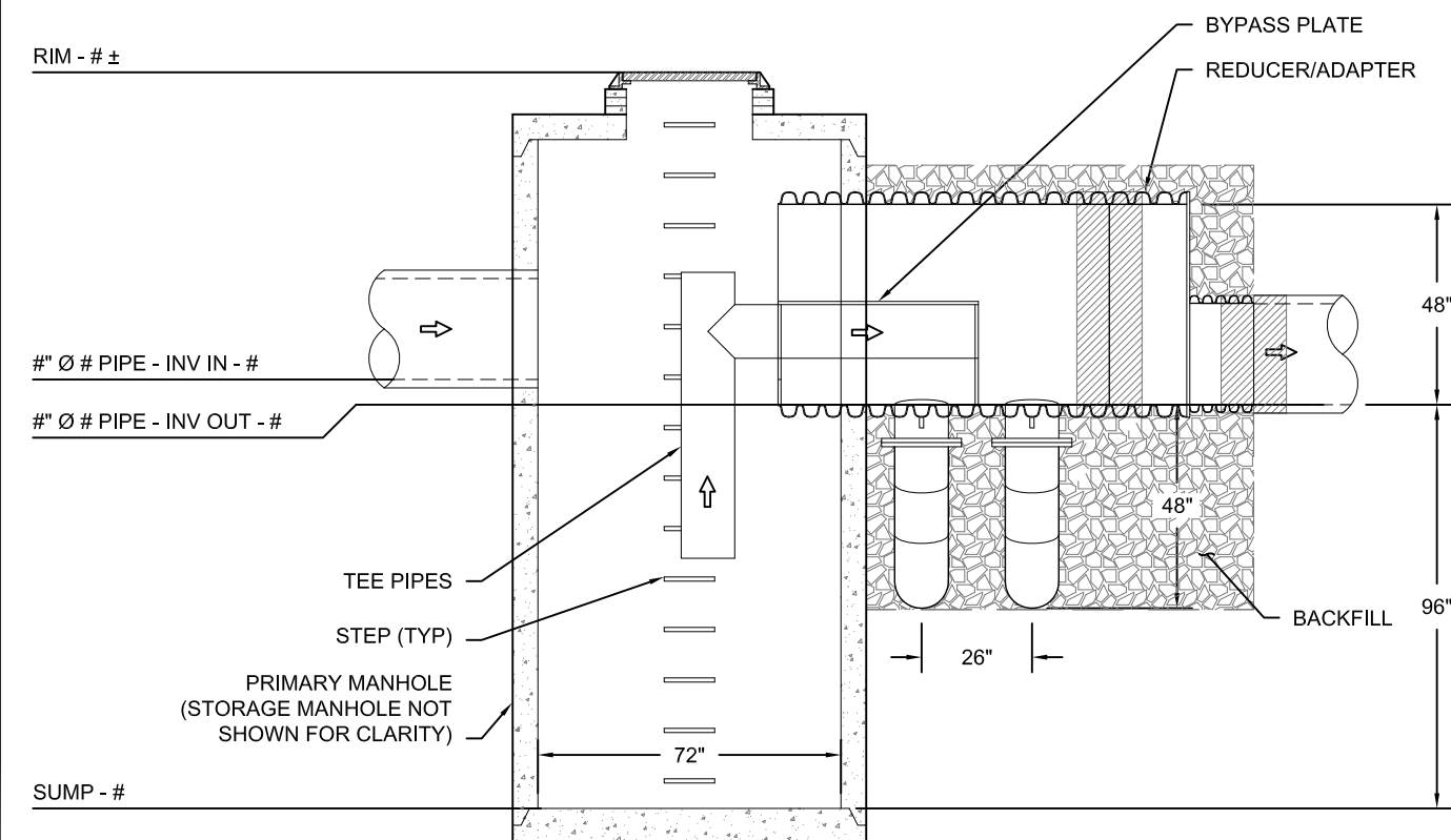
PROFILE A-A
